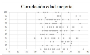
Figura 3. Correlación edad-mejoría.
